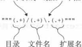
图 3.5 使用正则表达式将一个路径分割为目录、文件名和扩展名
