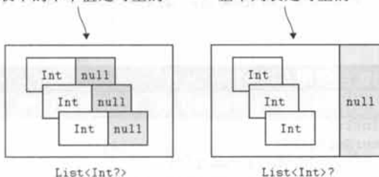
图 6.10 要小心决定什么是可空的：集合的元素还是集合本身？
