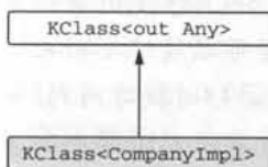
图 10.4 注解实参类型 CompanyImpl::class ( KClass<CompanyImpl> ) 是注解形参类型 ( KClass<out Any> ) 的子类型
