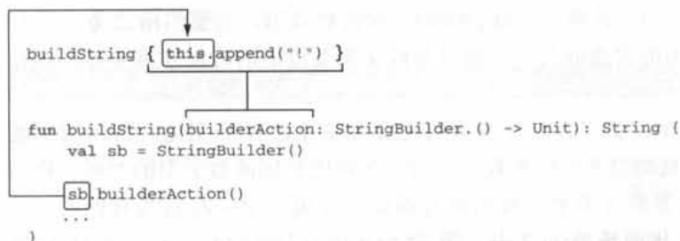
图 11.2 buildString 函数的实参（带接收者的 lambda）对应于扩展函数类型的形参（builderAction）。lambda 函数体被调用的时候接收者（sb）变成了一个隐式的接收者（this）
