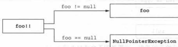
图 6.5 通过使用非空断言，如果值为 null，可以显式地抛出异常
